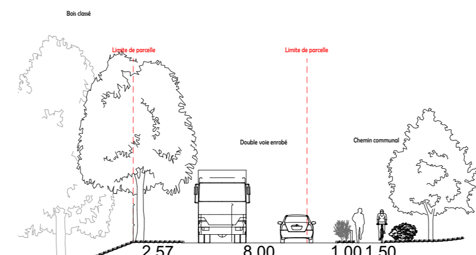
COUPE EE 1/200e
