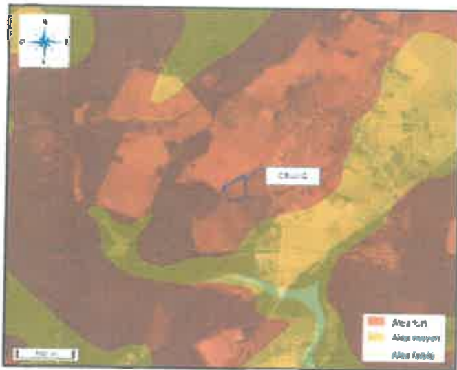
Figure 36 : Carte de l'aléa retrait-gonflement des argiles
