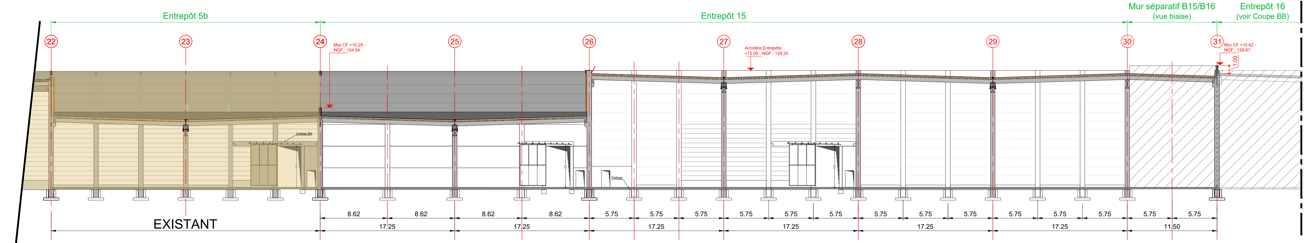
Coupe AA
